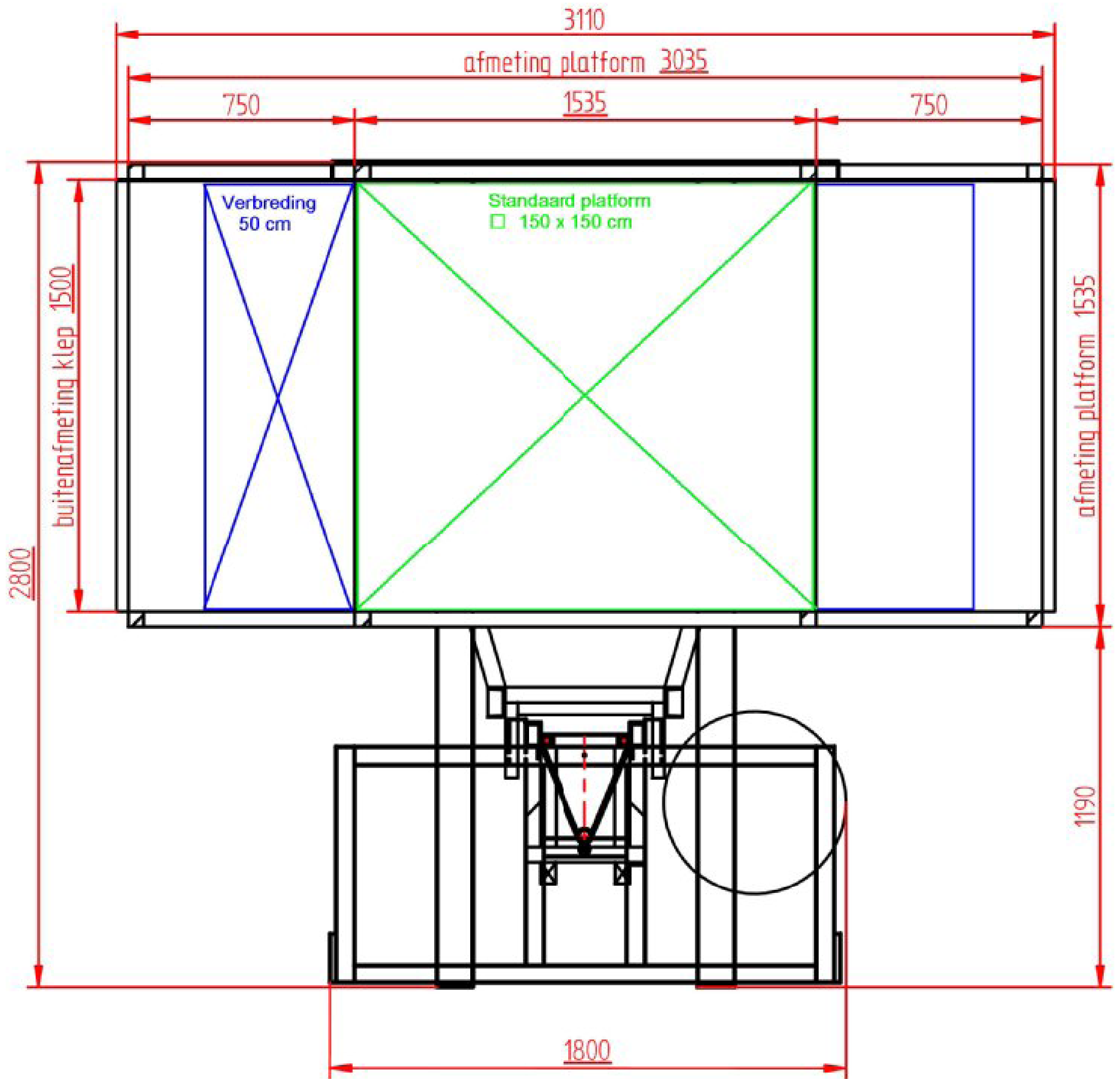
Bovenaanzicht
