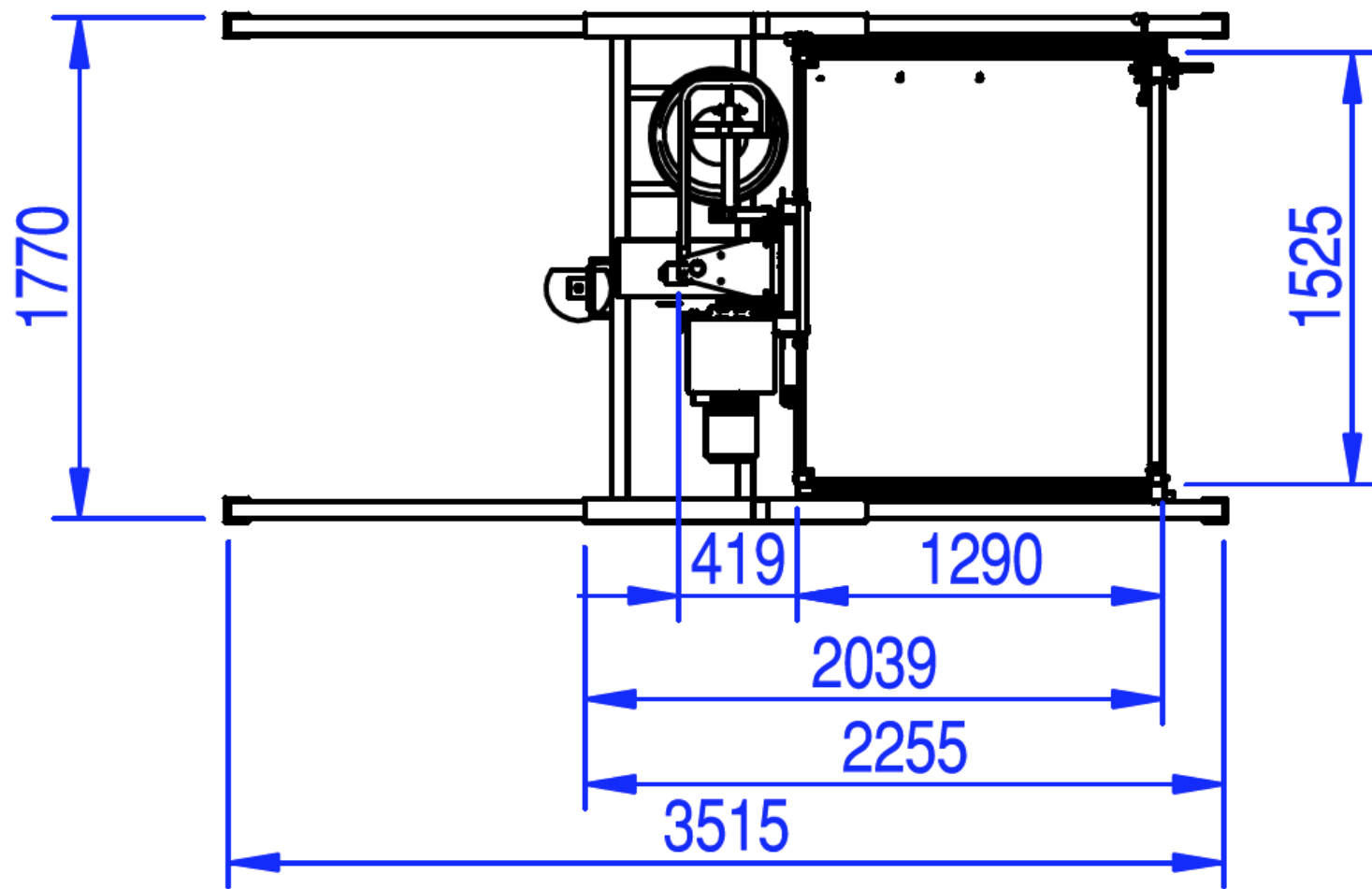
Bovenaanzicht
